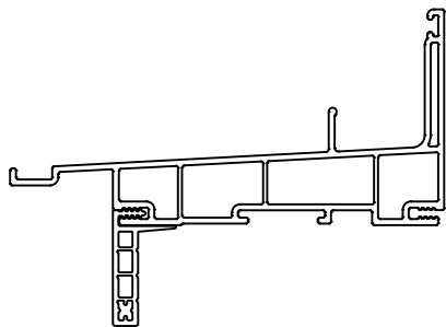
1" FLUSH FIN
