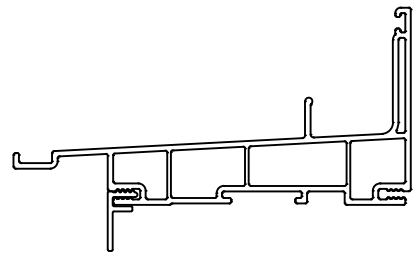
1/2" FLUSH FIN
