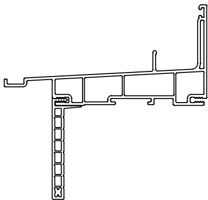
2" FLUSH FIN
